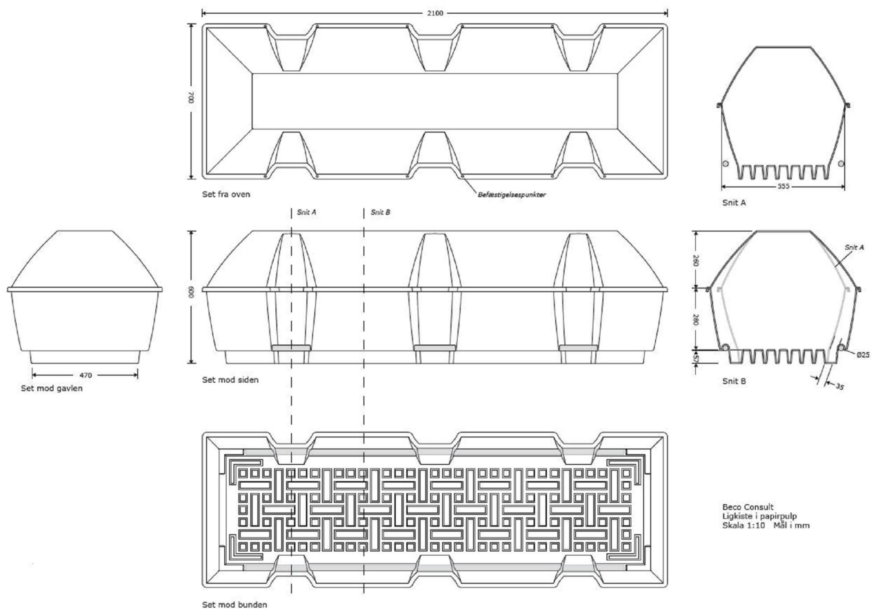
Figur 2: Tegning af kiste
